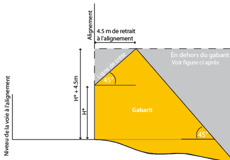
H* = Hauteur maximale autorisée à l'article 6
